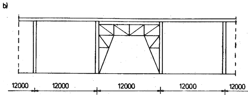
Schemat estakady z tężnikiem; a) tężnik krzyżowy, b) tężnik kratowy
