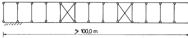
Schemat estakady z rozmieszczeniem tężników
