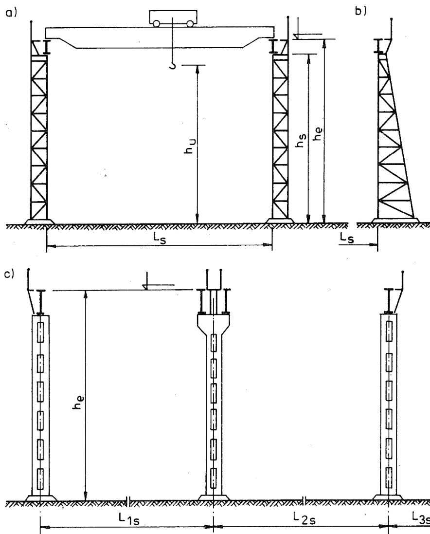
Schematy przekroju poprzecznego estakad suwnic pomostowych; a) estakada jednonawowa, b) słup estakady, c) estakada wielonawowa
